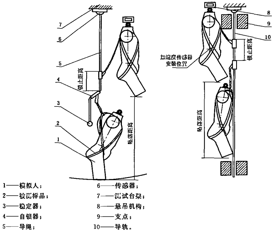
图 10 含安全绳、自锁器的坠落悬挂安全带的整体动态负荷测试示意图
