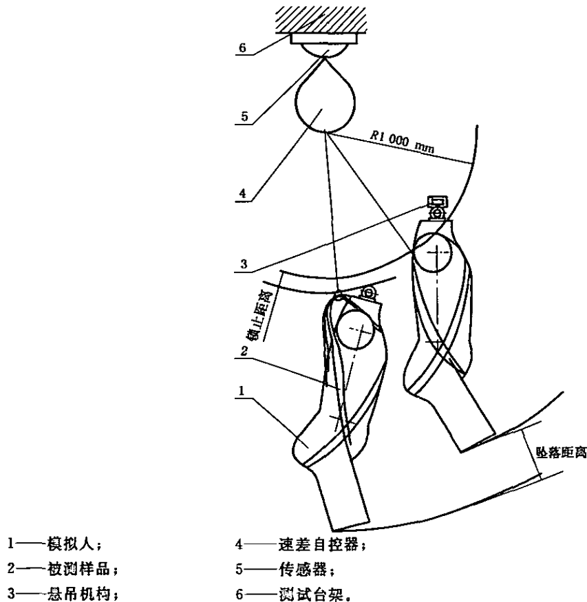
图 11 含速差自控器的坠落悬挂安全带的整体动态负荷测试示意图
