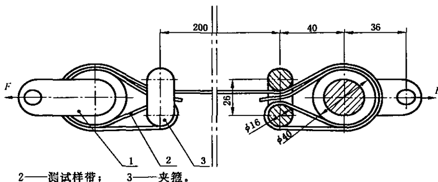
图 1 织带静态负荷测试夹具及夹持方法示意图
