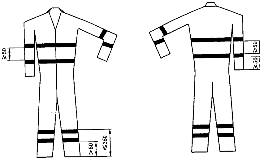
图 A.1 连裤工作服示意图
