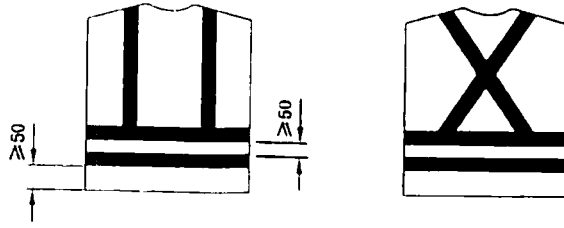
图 A.5 套头背心工作服示意图
