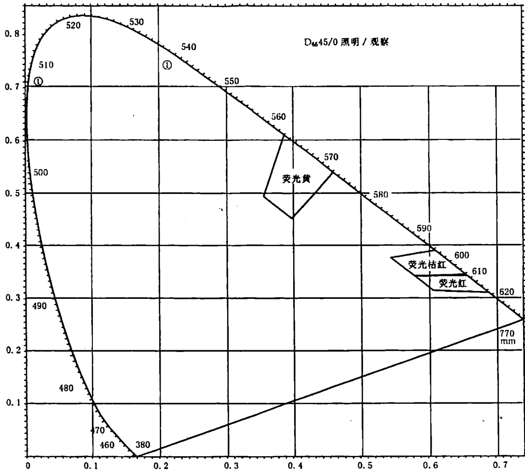
图 B.1 基底材料和组合材料色度图
